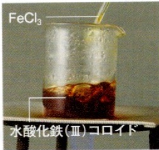
▲図23 水酸化鉄(Ⅲ)コロイド溶液
