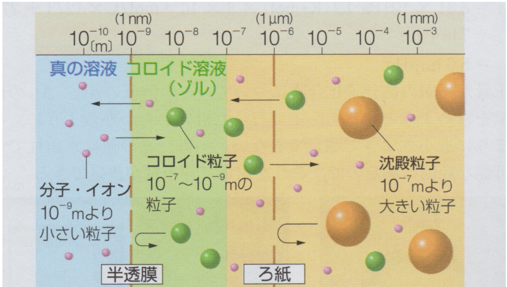
図 21 コロイド粒子の大きさ
