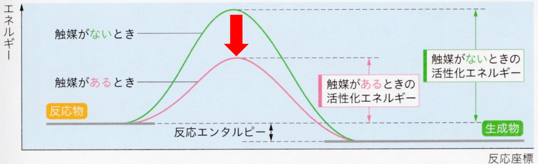
図 1 6 触媒の有無と活性化エネルギーの変化
